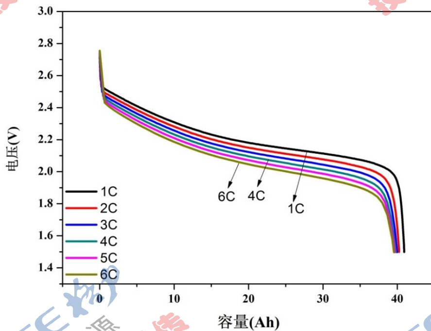
图 3 倍率放电性能曲线图 Fig.3 Rate discharge performance curve
